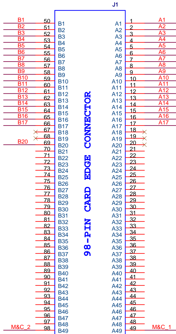
PCIe 98PIN Edge Conn
